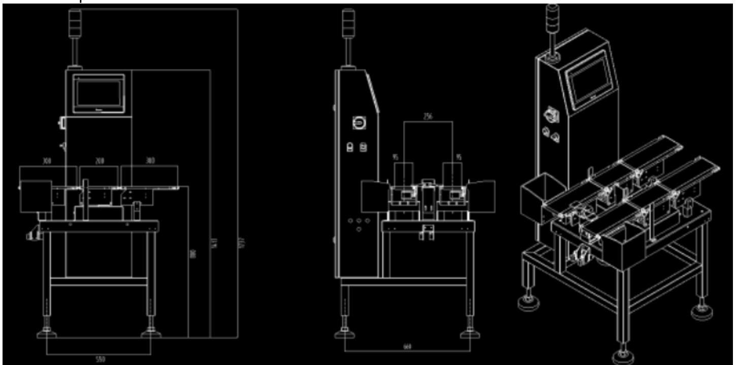
Máquina llenadora de polvo microdosificadora semiautomática HY900RT
